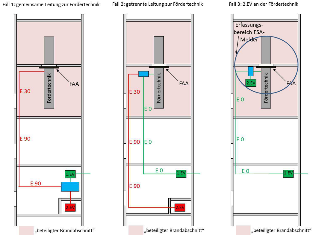
Abbildung 1: Energieversorgung FFS
